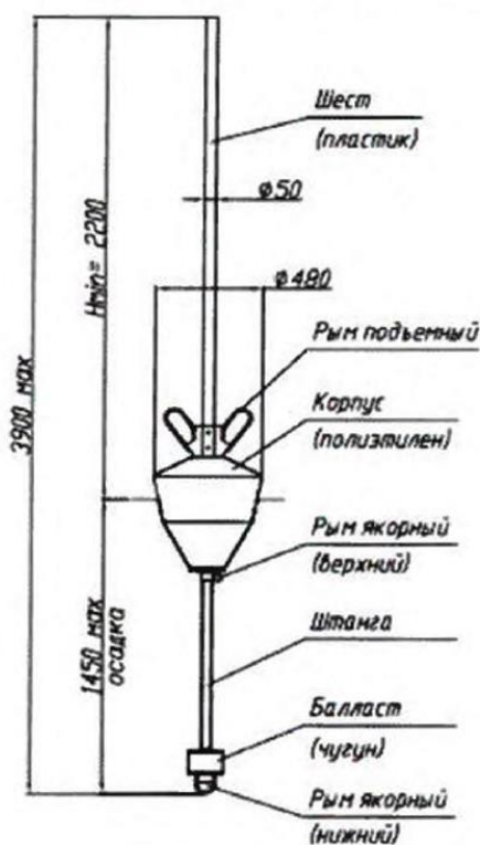
Рис. 3. Веха минная (тральная)
